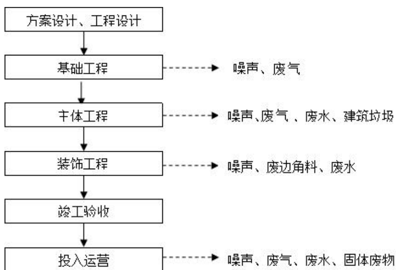
图 2.2-1 施工期工艺流程及产污环节图
