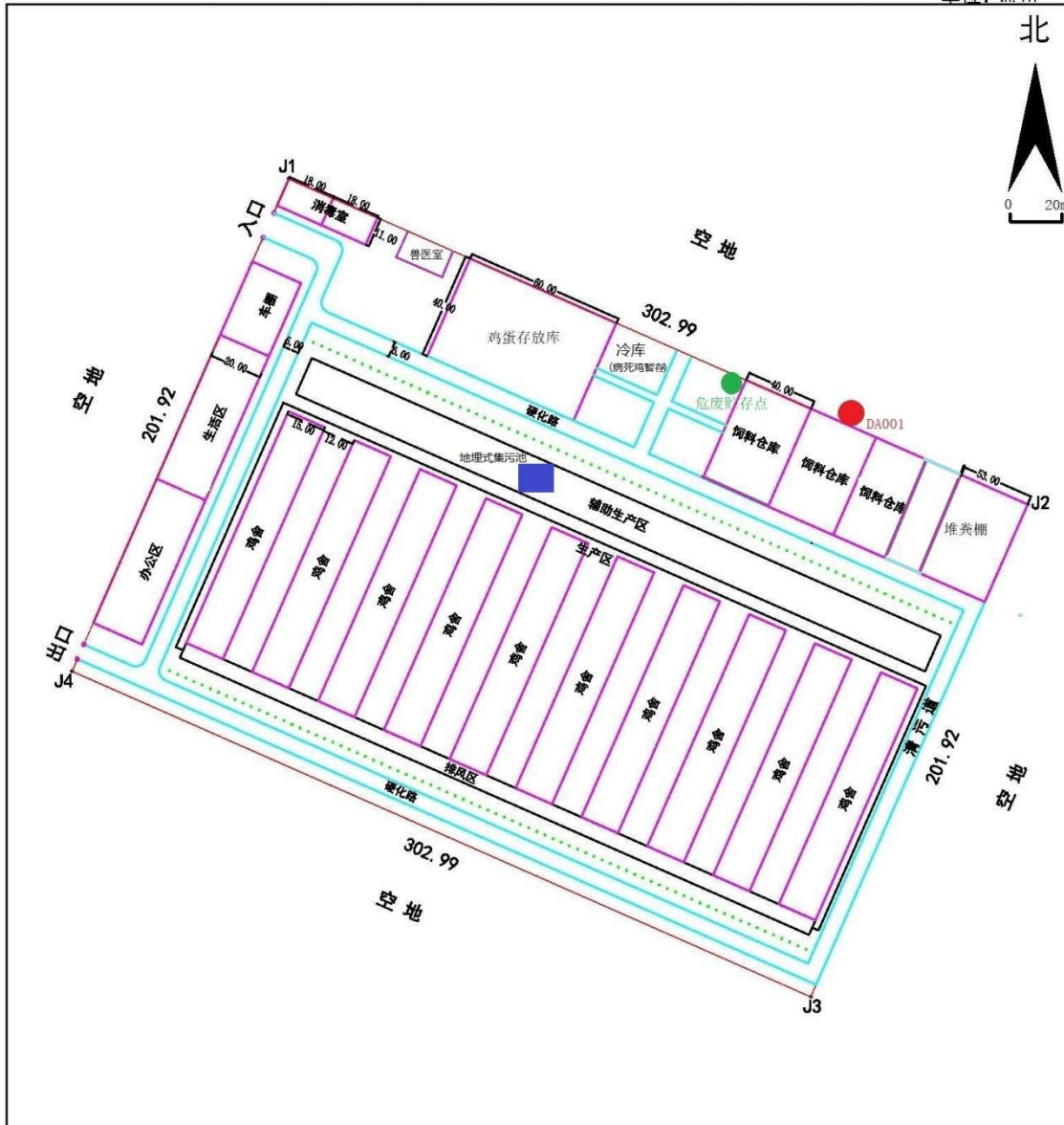
宣和镇汪园村蛋鸡养殖园区场区建设布局平面图
