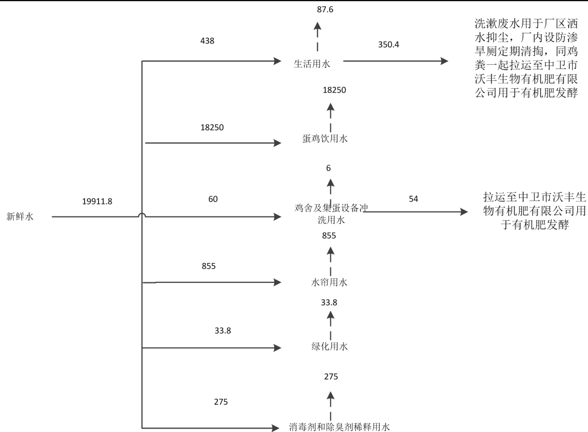
图 2.1-3 本项目水平衡图 单位：m³/a
